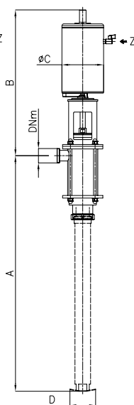
PA 140A - L con tubo de succión
