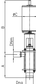
PA 140A - C
