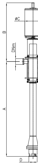
PA 140A - L con válvula de aspiración de fondo
